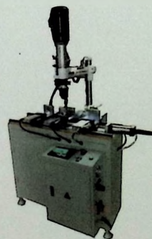
自动百页铣床
