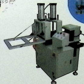
排料端面铣床
