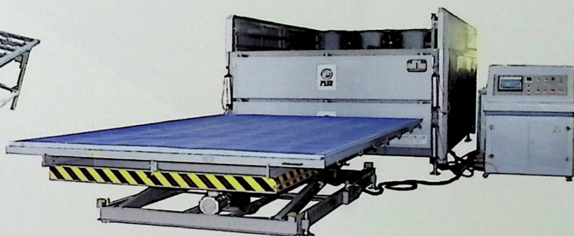
四层双循环设备
